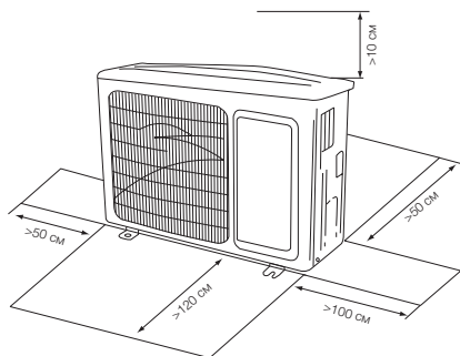
Размещение наружного блока относительно стен и потолка
