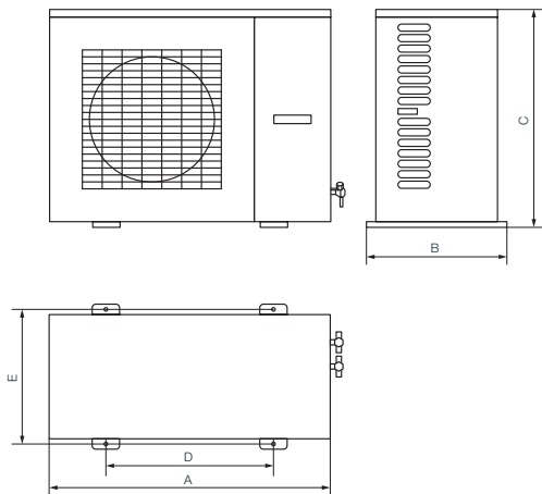
Размеры
